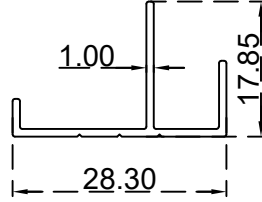
بروفيل ابواب ملتي لوك (17.85*28.3) ملم الرقم التسلسلي للصف: BLT740 الوزن 0.157:(Kg/m)
