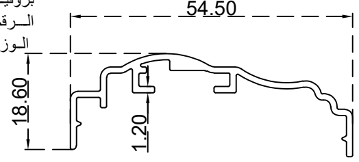
بروفيل ابواب ملتي لوك (18.6*54.5) ملم الرقم التسلسلي للصف: BLT976 الوزن 0.353:(Kg/m)
