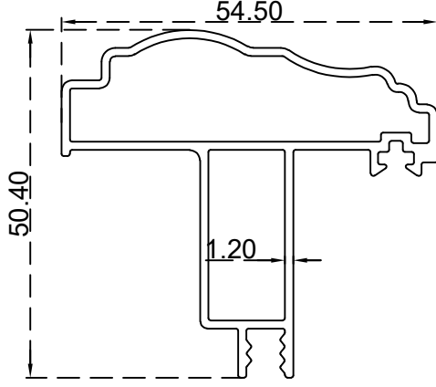
بروفيل ابواب ملتي لوك (50.4*54.5) ملم الرقم التسلسلي للصف: BLT974 الوزن 0.734:(Kg/m)
