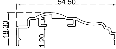
بروفيل ابواب ملتي لوك (18.3*54.5) ملم الرقم التسلسلي للصف: BLT975 الوزن 0.337:(Kg/m)
