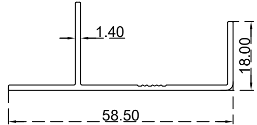
بروفيل ابواب ملتي لوك (18*58.5) ملم الرقم التسلسلي للصنف: BLT4594 الوزن 0.362:(Kg/m)
