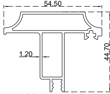
بروفيل ابواب تكني لوك (44.7*54.5) ملم الرقم التسلسلي للصنف: BLT3720 الوزن 0.746: (Kg/m)
