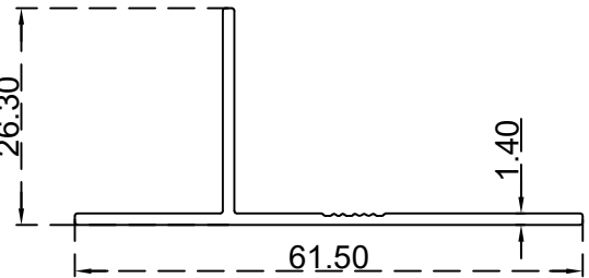
بروفيل ابواب ملتي لوك (26.3*61.5) ملم الرقم التسلسلي للصنف: BLT4593 الوزن 0.325:(Kg/m)
