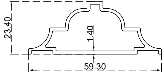
بروفيل ابواب ملتي لوك (23.4*59.3) ملم الرقم التسلسلي للصف: BLT754 الوزن 0.529:(Kg/m)
