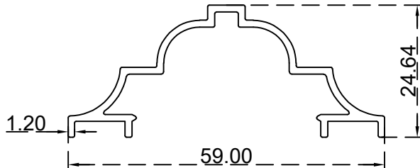
بروفيل ابواب ملتي لوك (24.64*59) ملم الرقم التسلسلي للصف: BLT1811 الوزن 0.395:(Kg/m)
