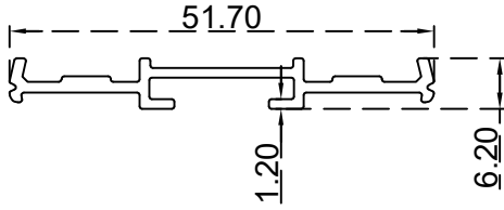
بروفيل ابواب ملتي لوك (6.20*51.7) ملم الرقم التسلسلي للصنف: BLT987 الوزن 0.282:(Kg/m)
