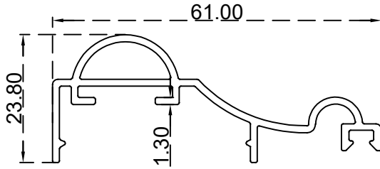
بروفيل ابواب ملتي لوك (23.8*61) ملم الرقم التسلسلي للصف: BLT1809 الوزن 0.501:(Kg/m)
