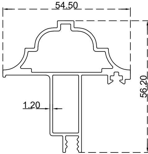
بروفيل ابواب تكني لوك (54.5*56.2) ملم الرقم التسلسلي للصنف: BLT3719 الوزن 1.105: (Kg/m)
