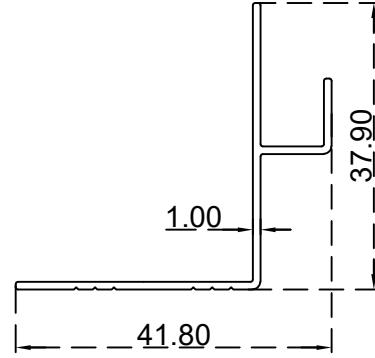
بروفيل ابواب ملتي لوك (37.9*41.8) ملم الرقم التسلسلي للصنف: BLT741 الوزن 0.236:(Kg/m)
