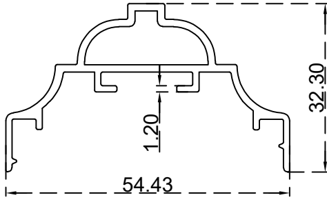
بروفيل ابواب تكني لوك (32.3*54.43) ملم الرقم التسلسلي للصنف: BLT3716 الوزن 0.543: (Kg/m)
