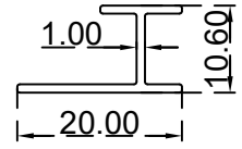
بروفيل ابواب ملتي لوك (10.6*20) ملم الرقم التسلسلي للصف: BLT743 الوزن 0.105:(Kg/m)
