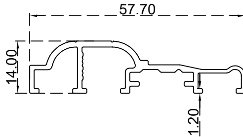
بروفيل ابواب متعدد الاقفال (14*57.7) ملم الرقم التسلسلي للصنف: BLT3339 الوزن 0.425: (Kg/m)
