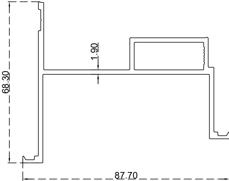
بروفيل ابواب ملتي لوك (68.3*87.7) ملم الرقم التسلسلي للصنف: BLT4600 الوزن 1.240:(Kg/m)
