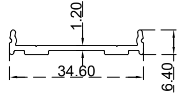
بروفيل ابواب ملتي لوك (6.4*34.6) ملم الرقم التسلسلي للصنف: BLT1810 الوزن 0.186:(Kg/m)
