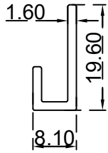
بروفيل ابواب ملتي لوك (8.10*19.6) ملم الرقم التسلسلي للصف: BLT739 الوزن 0.142:(Kg/m)
