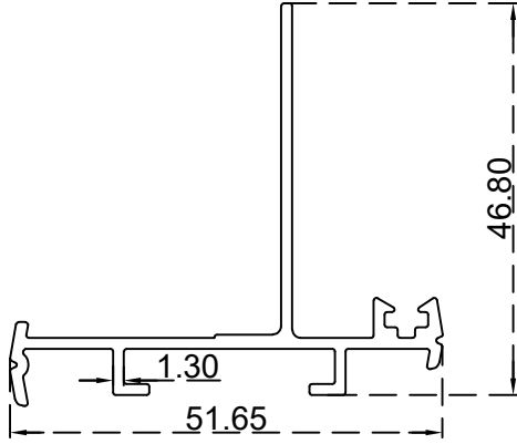
بروفيل ابواب ملتي لوك (46.8*51.65) ملم الرقم التسلسلي للصنف: BLT982 الوزن 0.487:(Kg/m)
